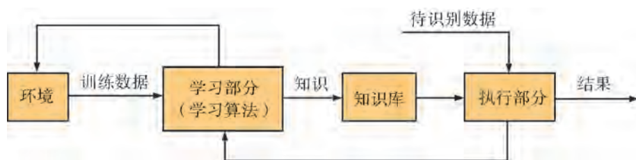
图6-9 训练模型程序的逻辑结构
