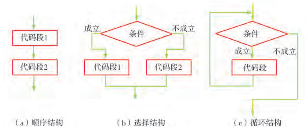
图3-9 三种基本控制结构
