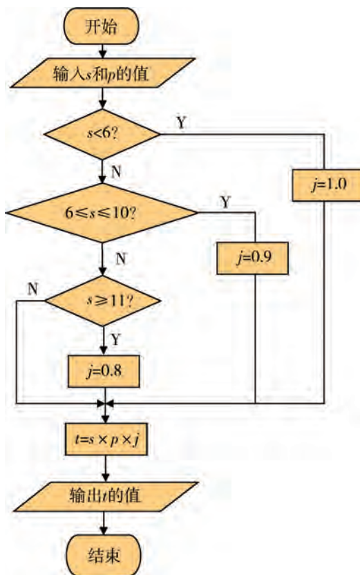
图4-8 网购笔记本的金额计算流程图
