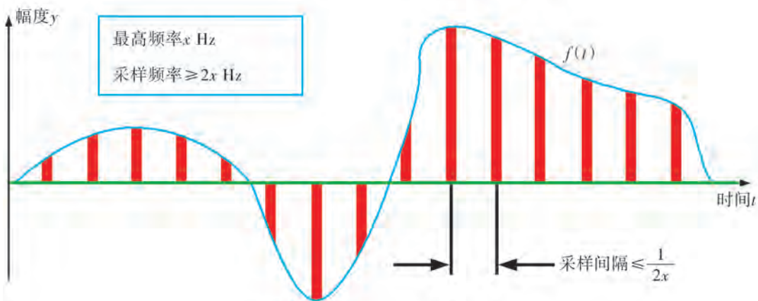
图1-11 奈奎斯特采样定理示意图
