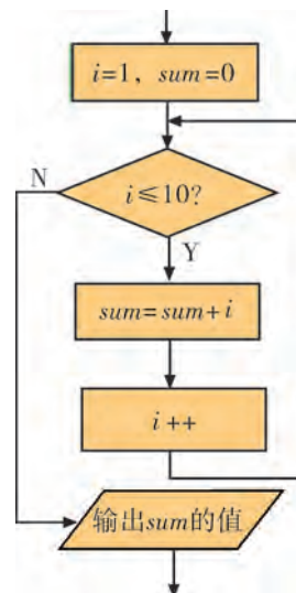
图4-14 累加算法流程图
