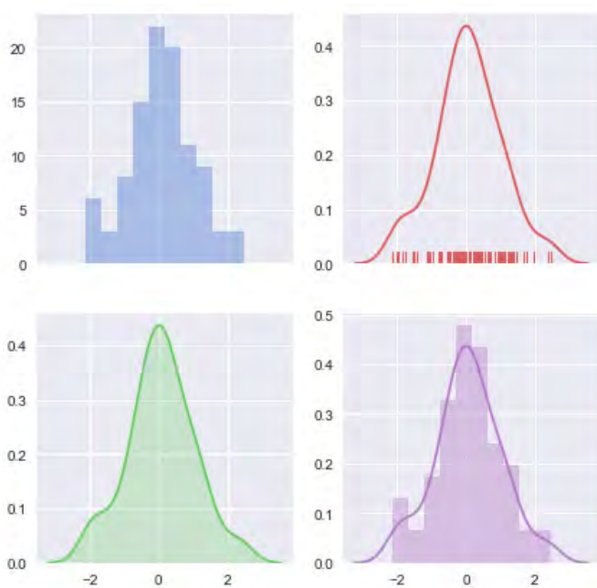
图5-13 直方图程序5-7
