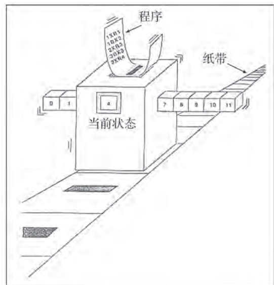
图1-14 图灵机模型
