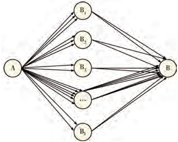
图3-4 从A市经 B_1, B_2, \dots, B_k 市到B市的交通情况
