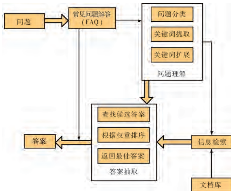
图6-5 典型的智能问答系统结构示意图
