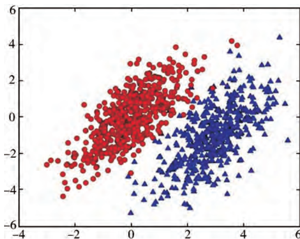
图5-11 数据分布
