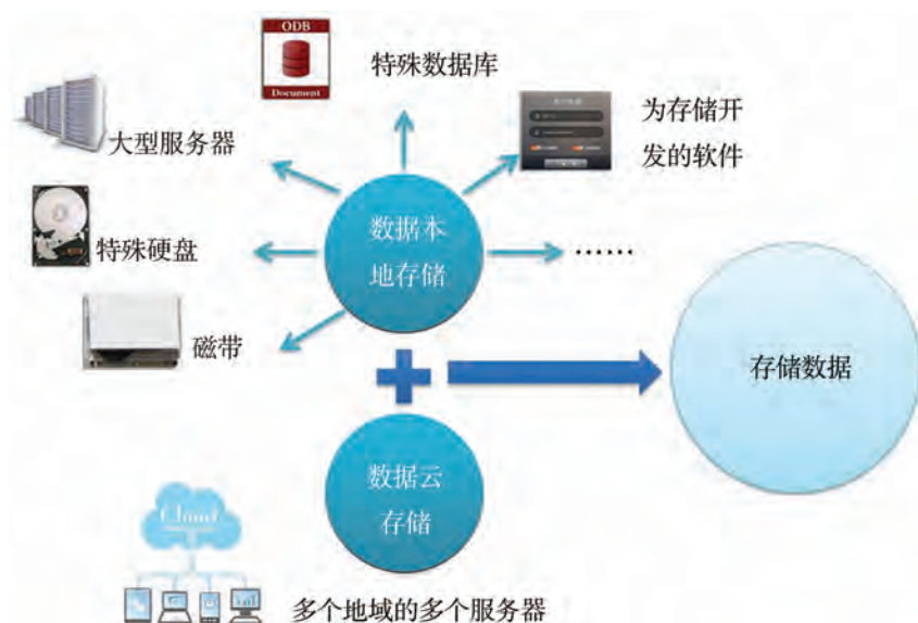
图5-6 数据的存储
