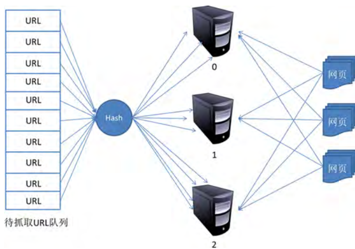
图5-4 网络爬虫
