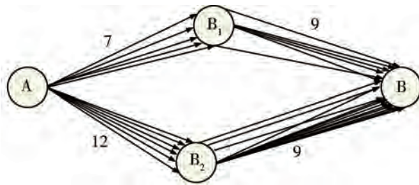
图3-5 从A市到B市的班次状况
