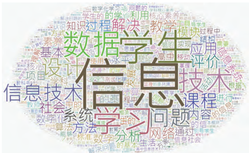
图5-12 词云图
