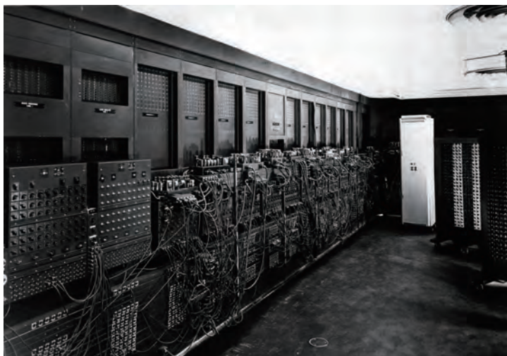
图3-17 计算机ENIAC
