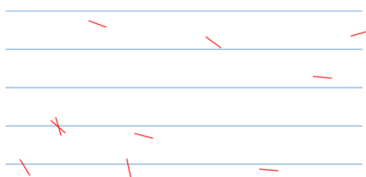
图2-10 投针实验
